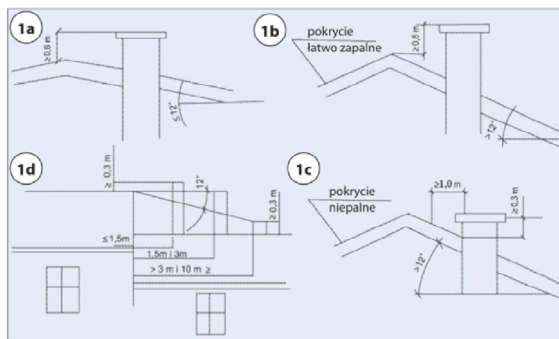
Rys. 1 Usytuowanie wylotów kominia
